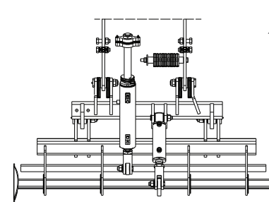
ASSIEME LATO SINISTRO (VISTA IN PIANTA) LEFT SIDE ASSEMBLY (PLAN VIEW)
