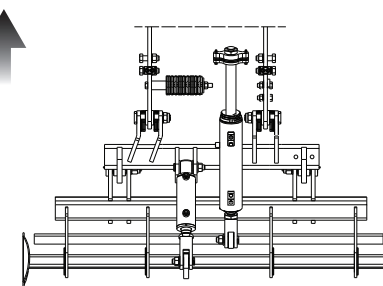
ASSIEME LATO DESTRO (VISTA IN PIANTA) RIGHT SIDE ASSEMBLY (PLAN VIEW)
