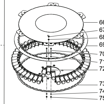
VERSIONE 48 USCITE 48 OUTPUTS VERSION
